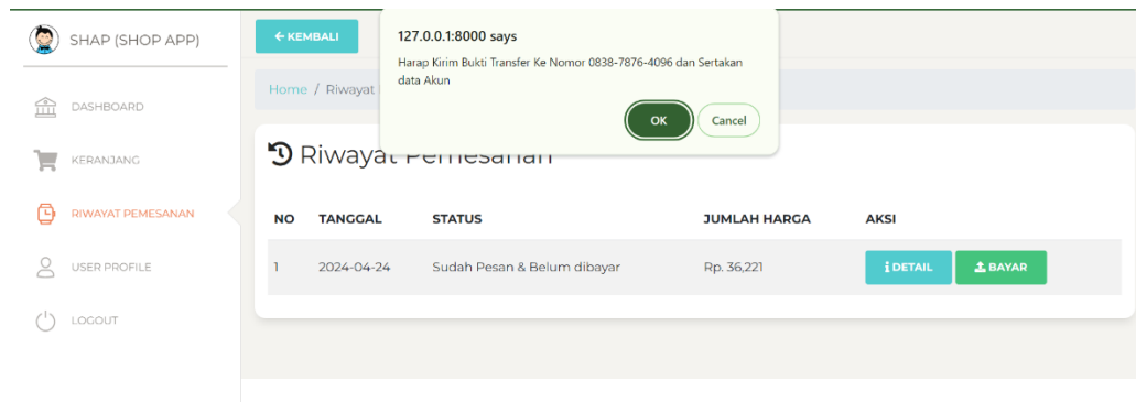
Gambar 10 Riwayat Pemesanan.
