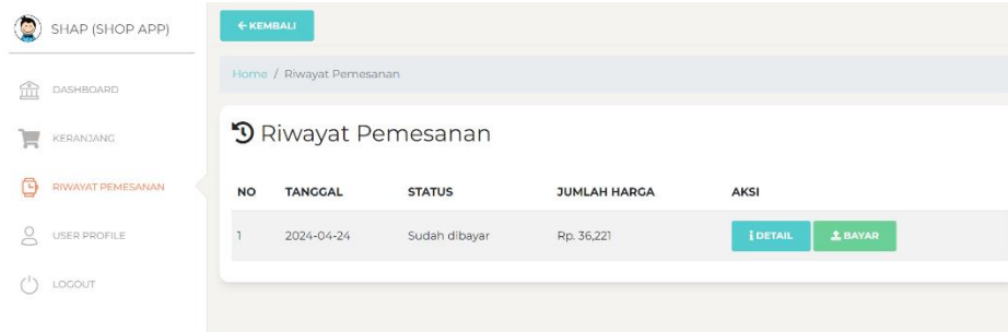
Gambar 20 Riwayat Pemesanan
