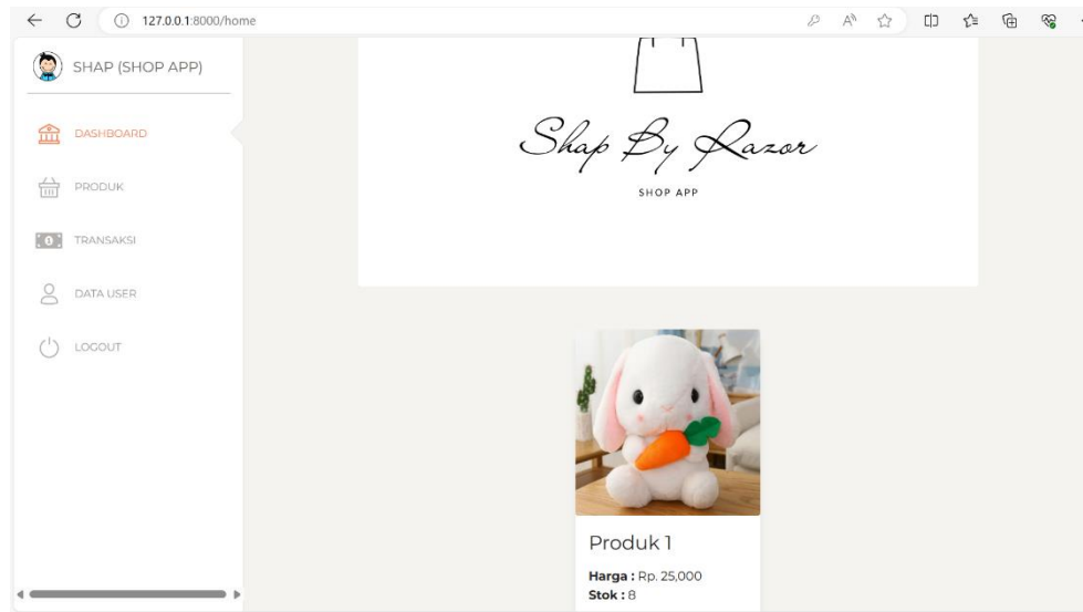
Gambar 2 Halaman Utama
