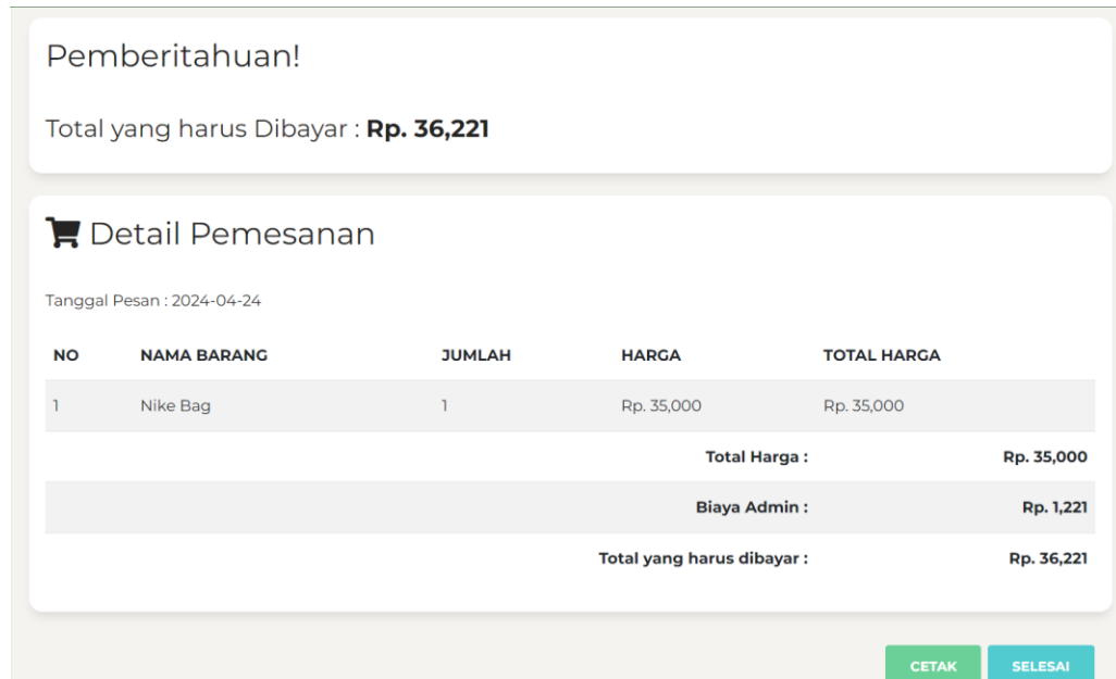
Gambar 8 Detail Pesanan.
