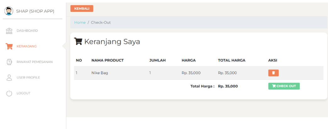
Gambar 7 Halaman Keranjang.
