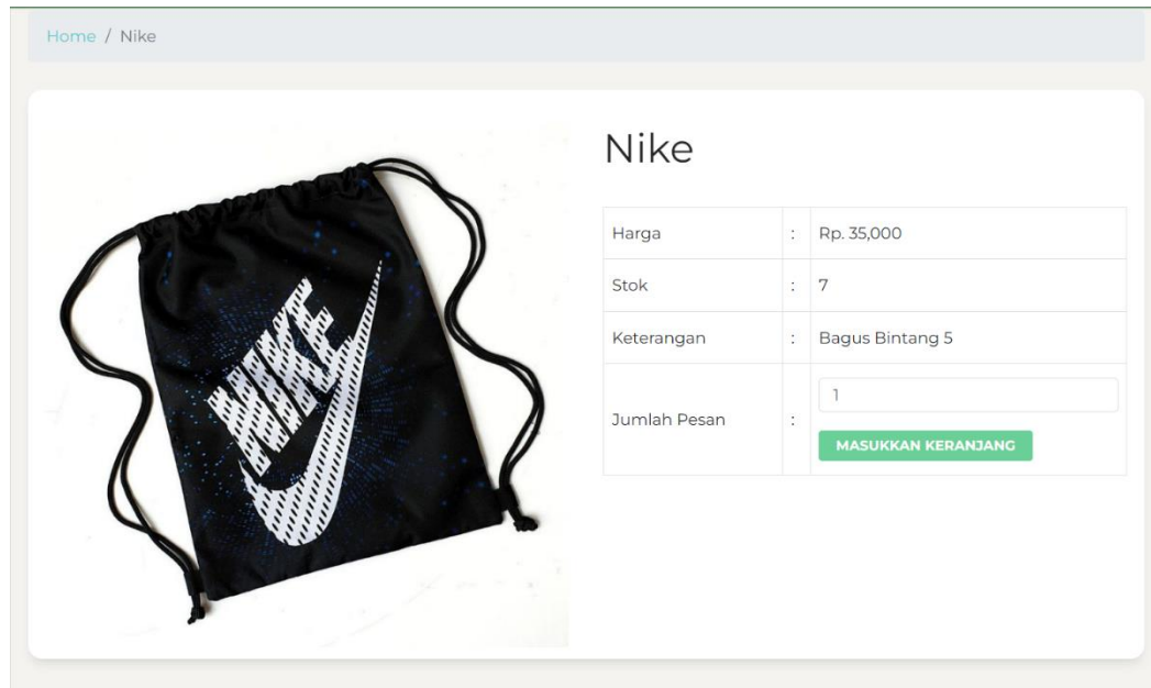
Gambar 6 Pesan.
